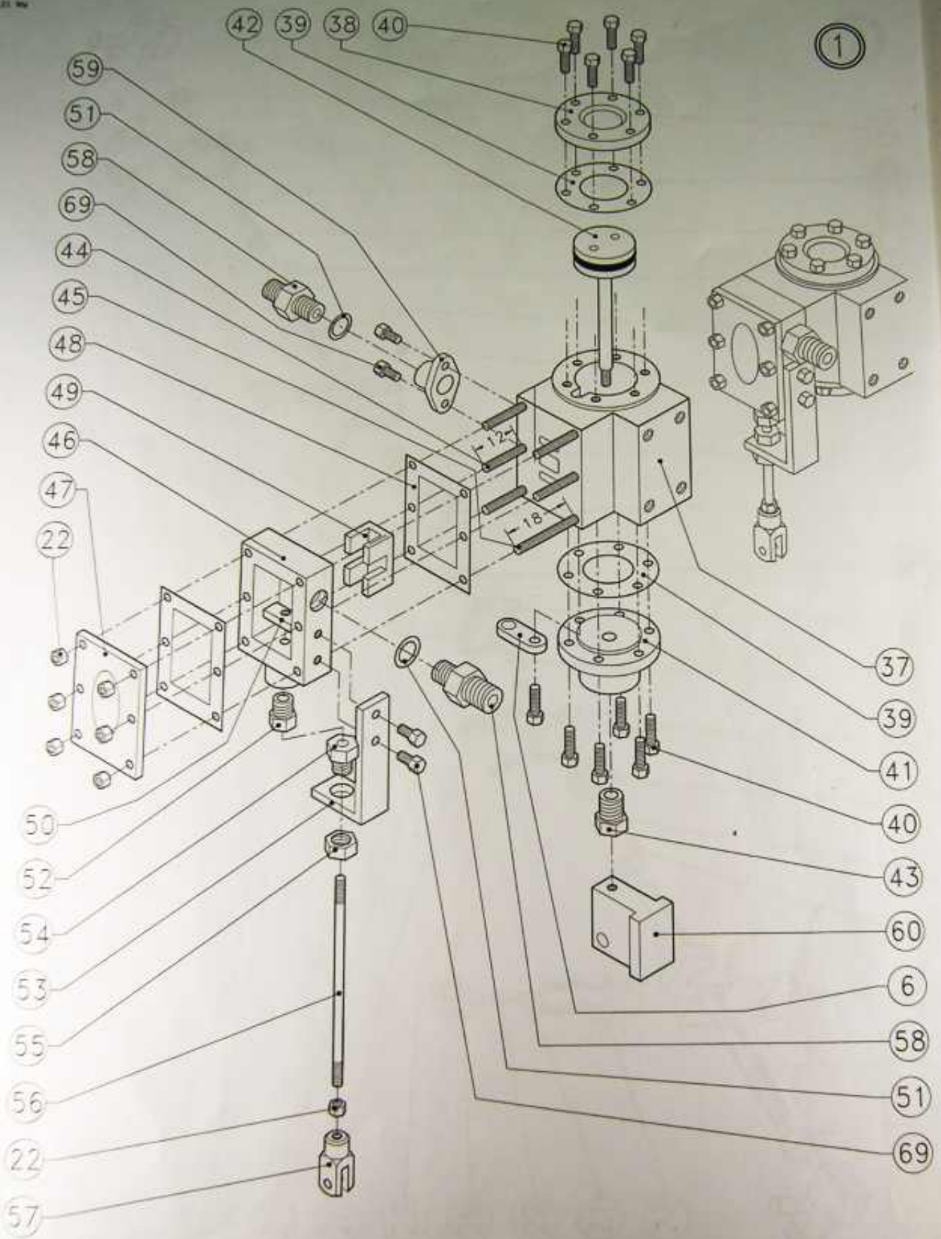
REGNER Aurach - "Neptun" - Zylinder
